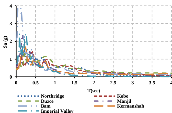
شکل ۸- شتاب‌نگاشت‌های مقیاس‌شده
