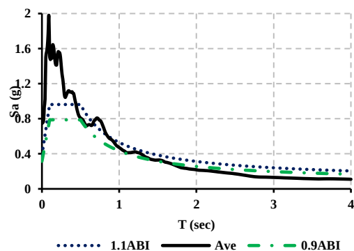
شکل ۷- مقایسه نمودار متوسط با ASCE7-22
